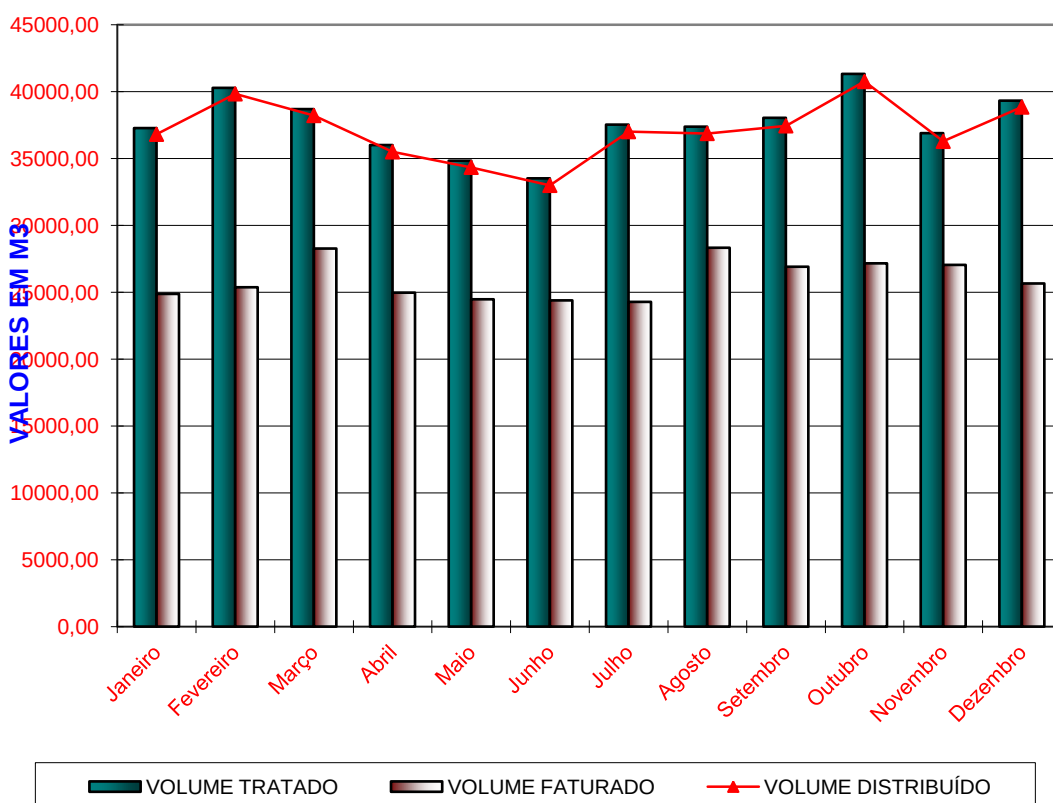
REPRESENTAÇÃO GRÁFICA DOS VOLUMES TRATADO, FATURADO E DISTRIBUÍDO
