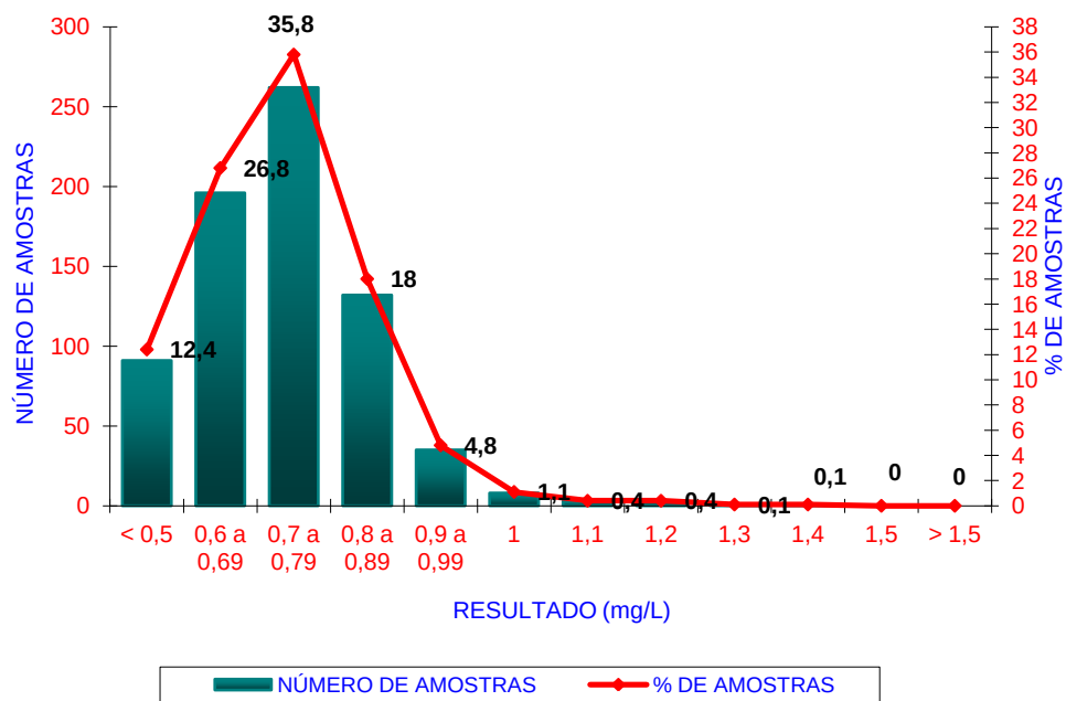
HISTOGRAMA DOS RESULTADOS DAS ANÁLISES DE ÍON FLUORETO REALIZADAS NO ANO DE 2006
