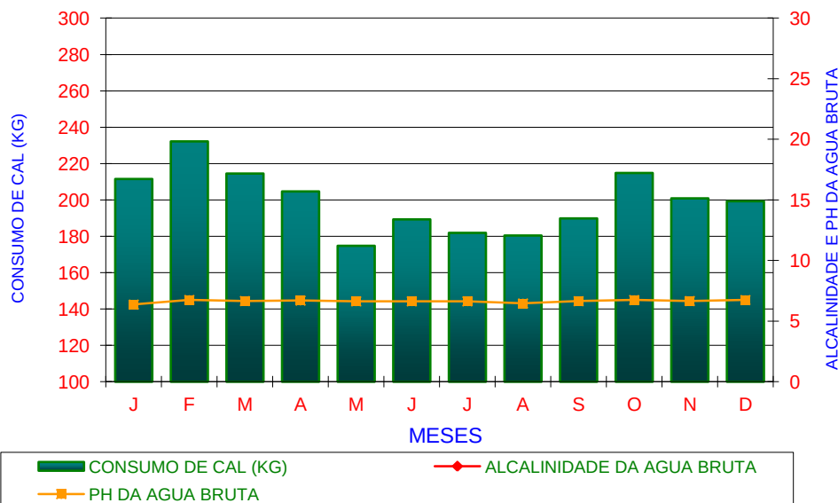
REPRESENTAÇÃO GRÁFICA DO CONSUMO DE CAL (KG) EM RELAÇÃO AO PH DA AGUA BRUTA
