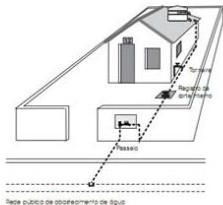
Figura 2 - Modelos de Locais para Instalação da Caixa Padrão de Hidrômetros
