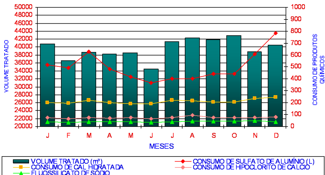
REPRESENTAÇÃO GRÁFICA DO VOLUME TRATADO COM CONSUMO DE PRODUTOS QUÍMICOS
