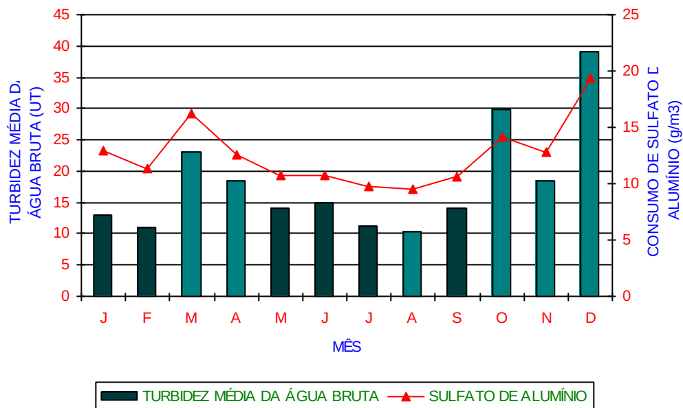
REPRESENTAÇÃO GRÁFICA DA TURBIDEZ MÉDIA DA ÁGUA BRUTA RELACIONADA COM CONSUMO DE SULFATO DE ALUMÍNIO
