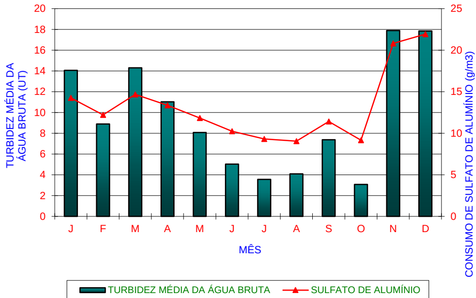
REPRESENTAÇÃO GRÁFICA DA TURBIDEZ MÉDIA DA ÁGUA BRUTA RELACIONADA COM CONSUMO DE SULFATO DE ALUMÍNIO
